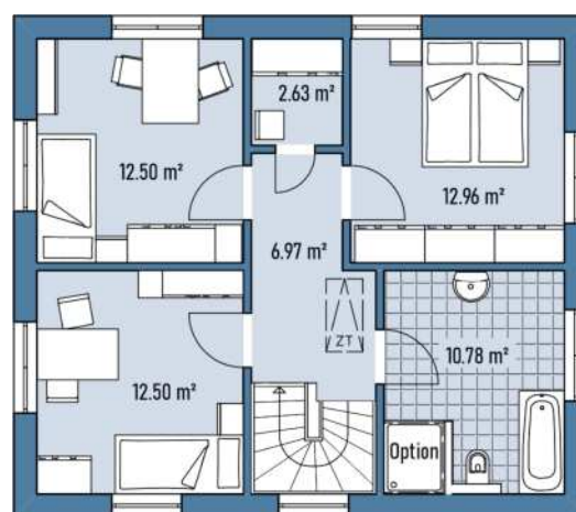
Grundriss DG
