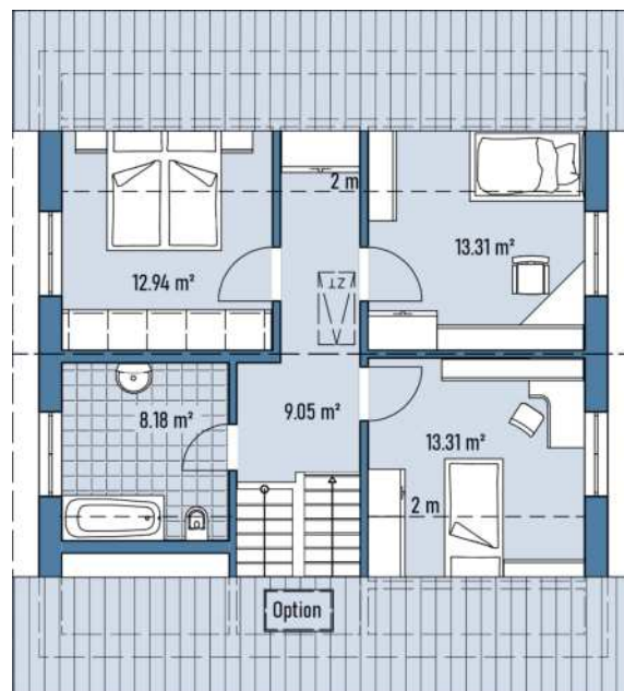
Grundriss DG
