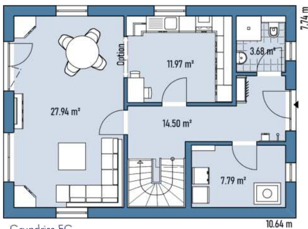
Grundriss EG
