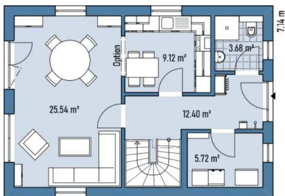
Grundriss EG
