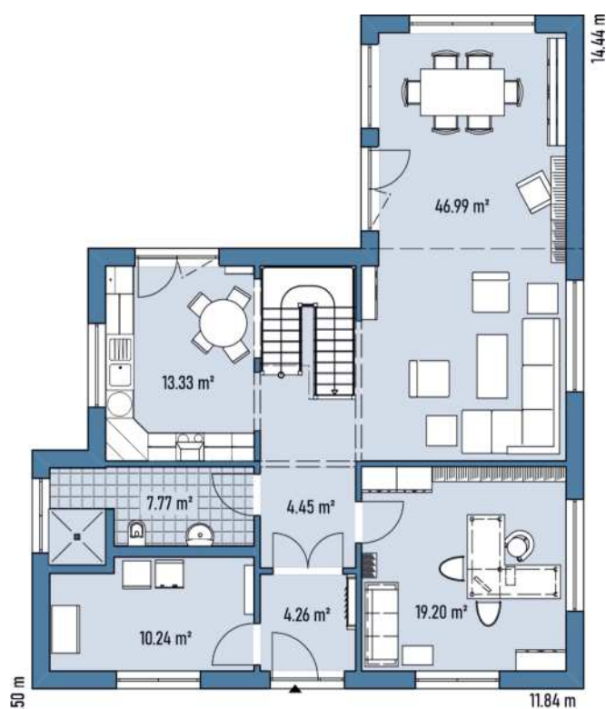
Grundriss EG
