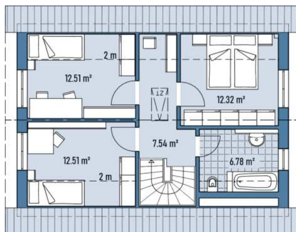
Grundriss DG
