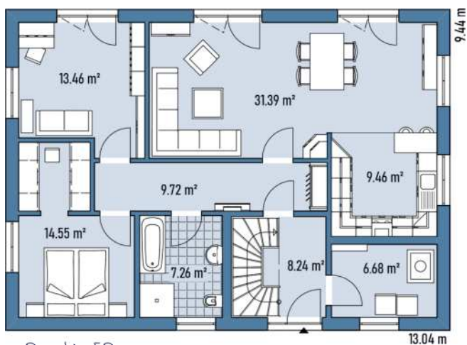
Grundriss EG
