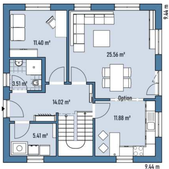
Grundriss EG
