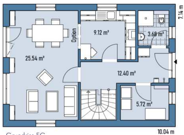
Grundriss EG
