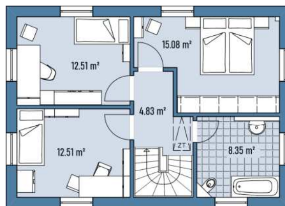
Grundriss DG
