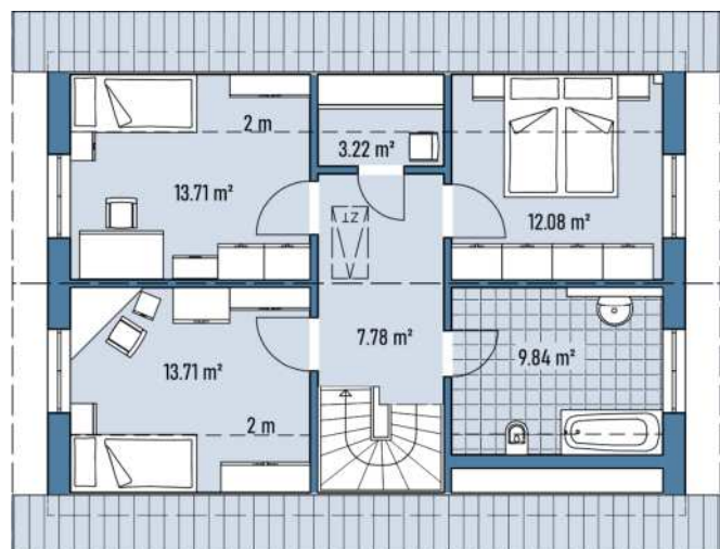
Grundriss DG
