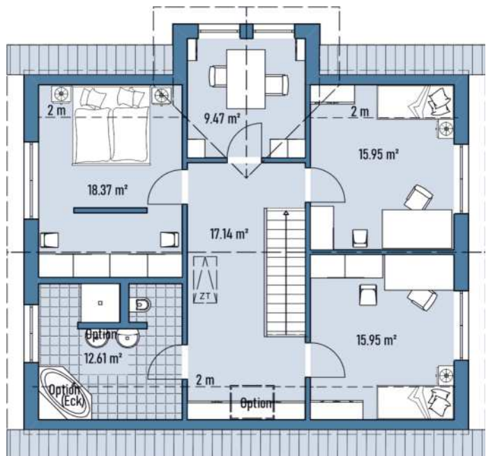
Grundriss DG
