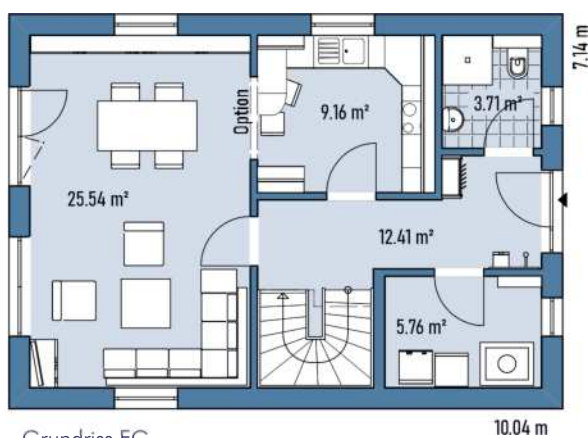
Grundriss EG
