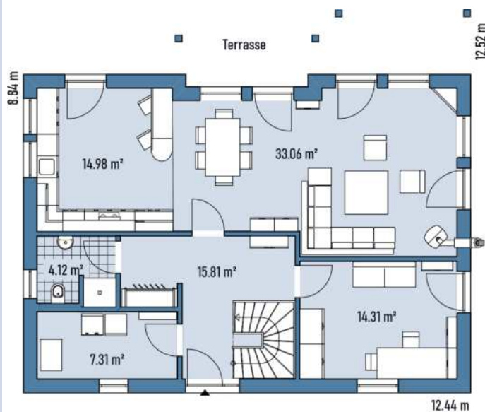
Grundriss EG
