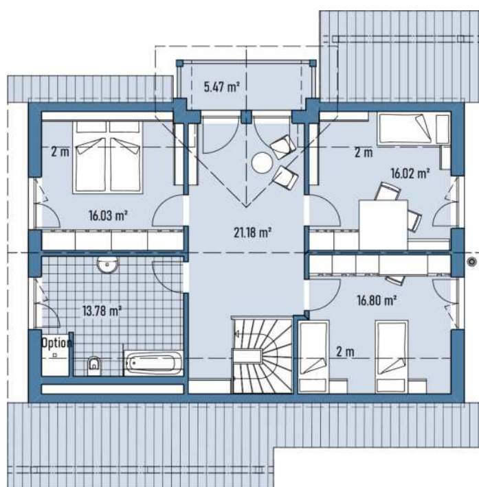
Grundriss DG
