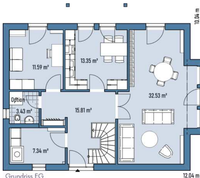
Grundriss EG
