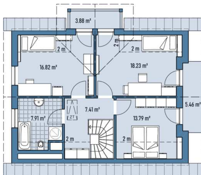
Grundriss DG
