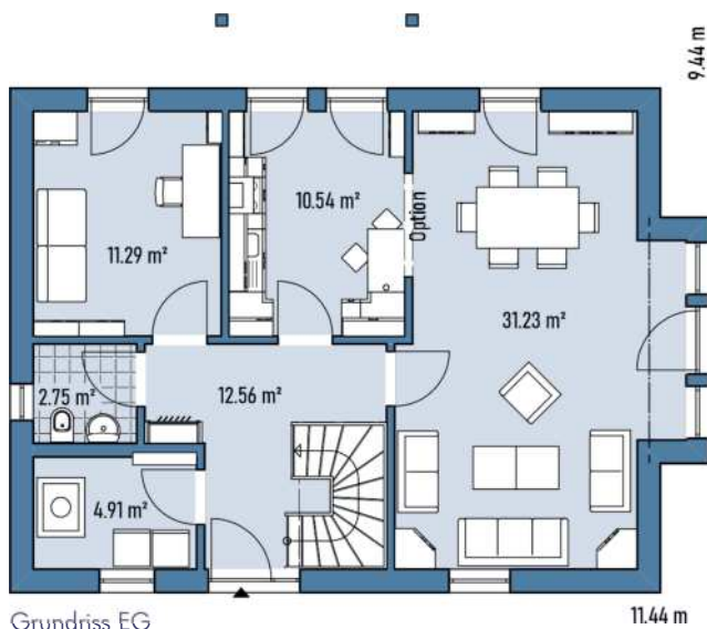
Grundriss EG
