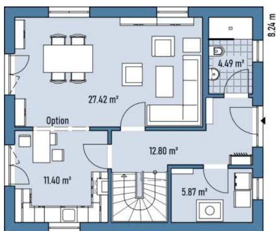
Grundriss EG
