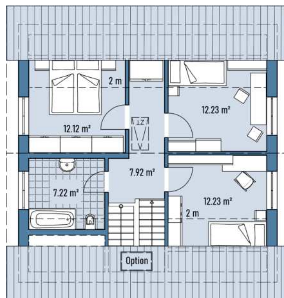
Grundriss DG
