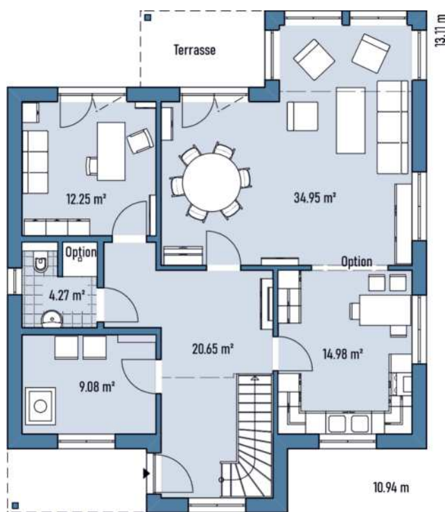
Grundriss EG
