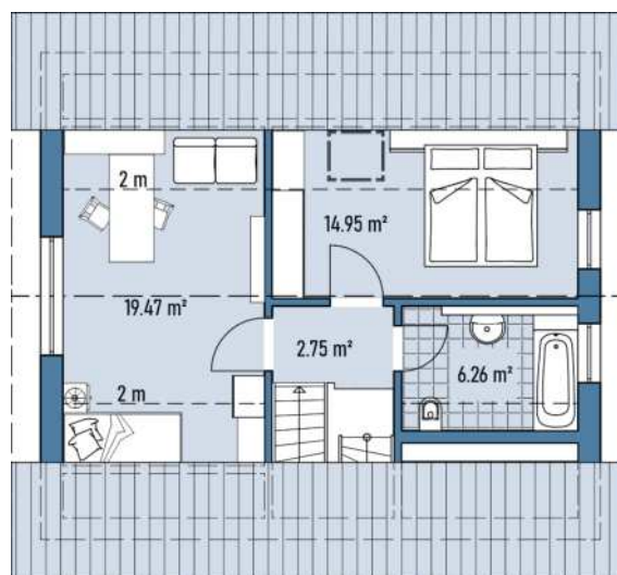
Grundriss DG
