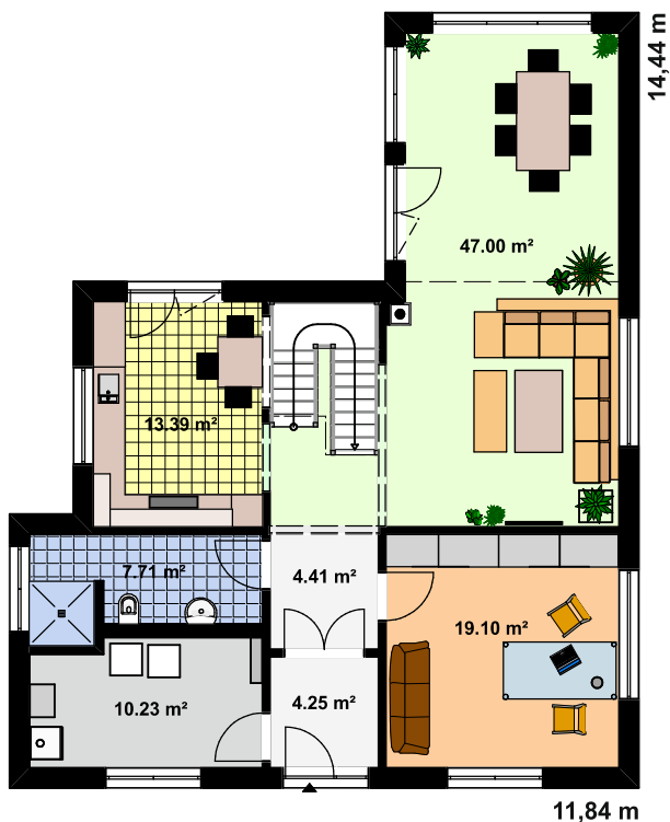
Grundriss Erdgeschoss
