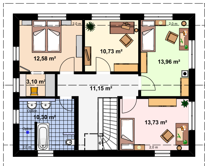
Grundriss Dachgeschoss
