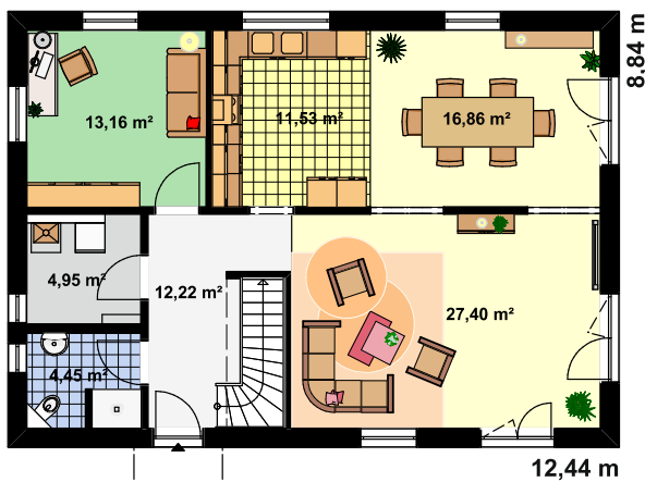
Grundriss Erdgeschoss
