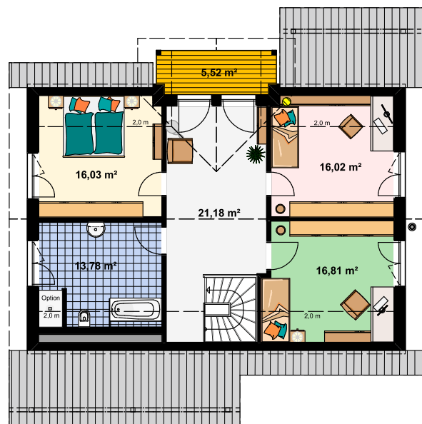
Grundriss Dachgeschoss
