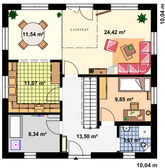
Grundriss Erdgeschoss
