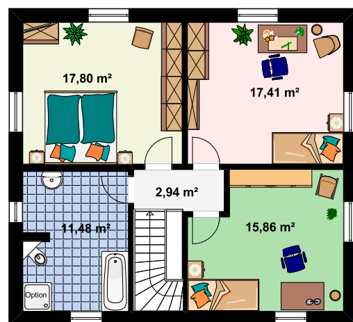
Grundriss Dachgeschoss
