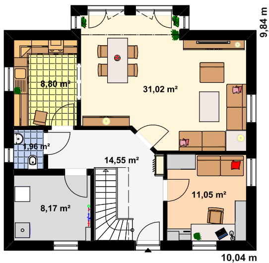
Grundriss Erdgeschoss
