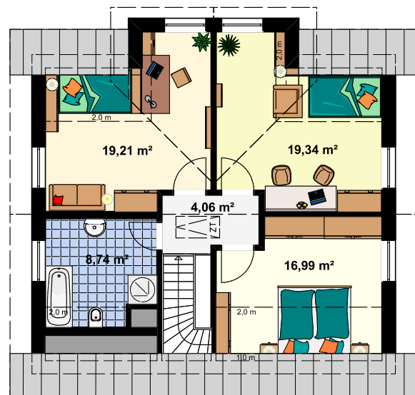
Grundriss Dachgeschoss
