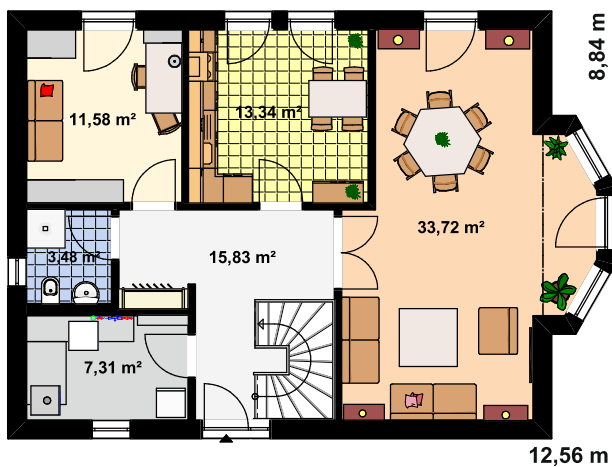
Grundriss Erdgeschoss
