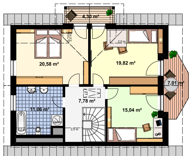
Grundriss Dachgeschoss
