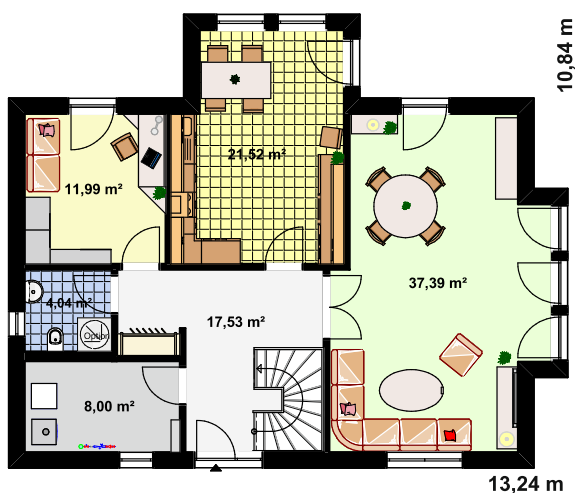
Grundriss Erdgeschoss
