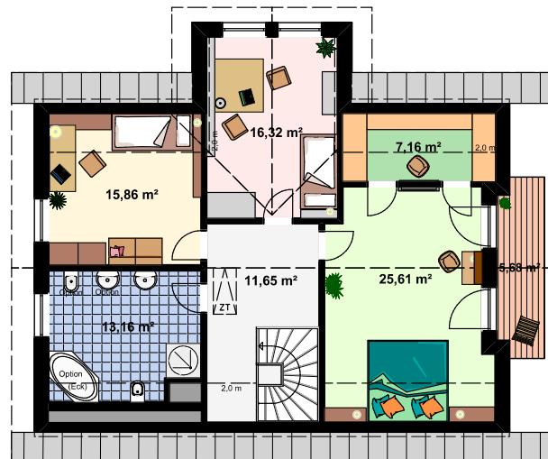
Grundriss Dachgeschoss
