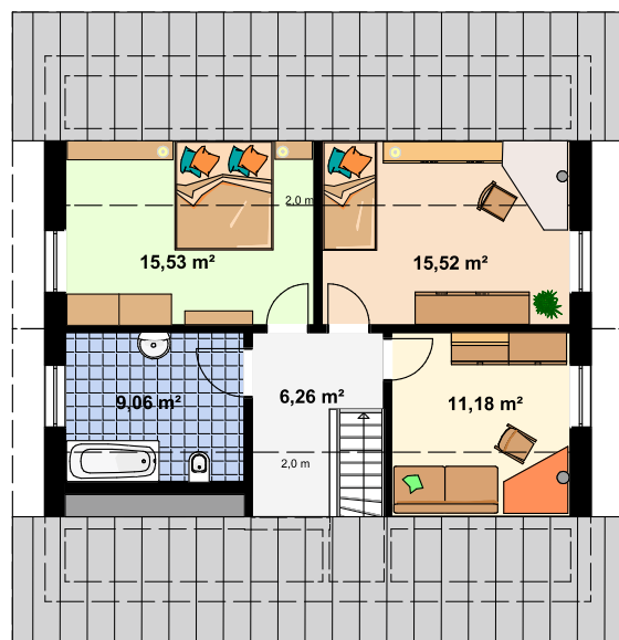
Grundriss Dachgeschoss
