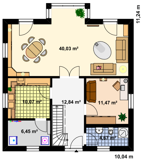
Grundriss Erdgeschoss
