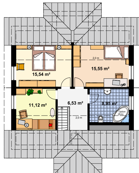
Grundriss Dachgeschoss
