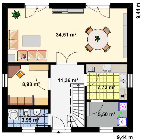
Grundriss Erdgeschoss
