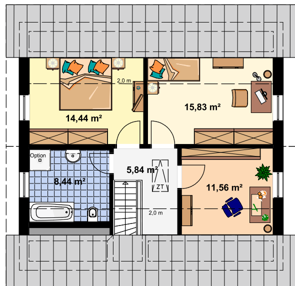
Grundriss Dachgeschoss
