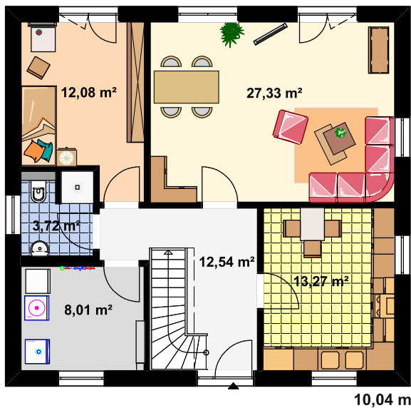
Grundriss Erdgeschoss
