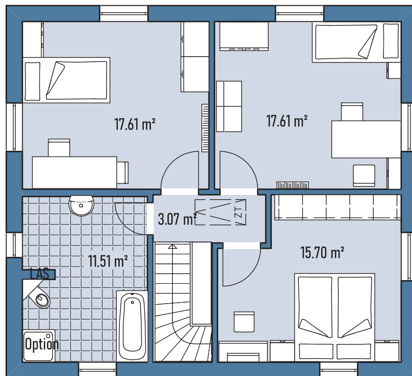
Grundriss DG
