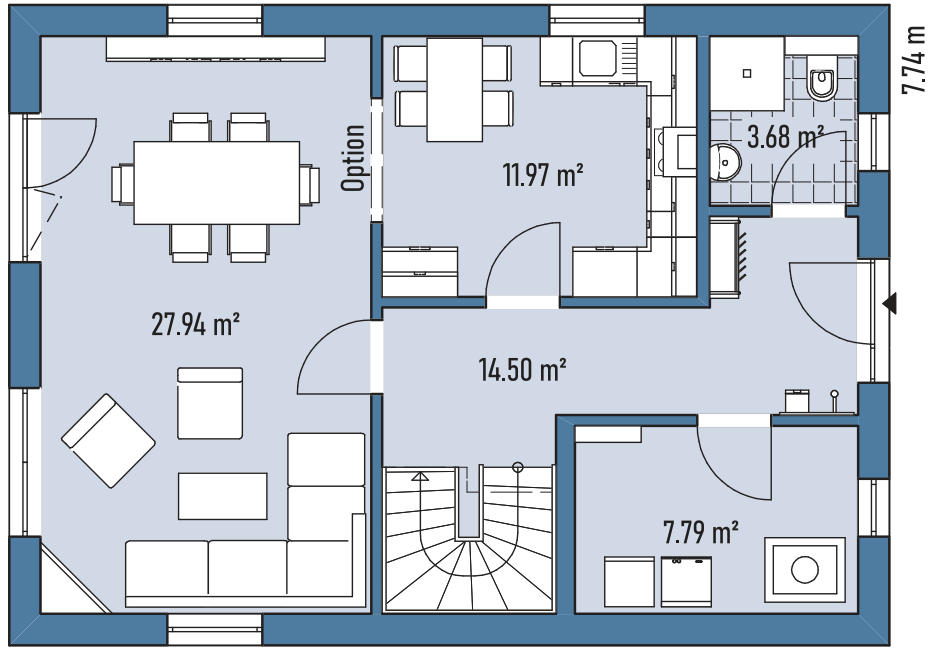
Grundriss EG
