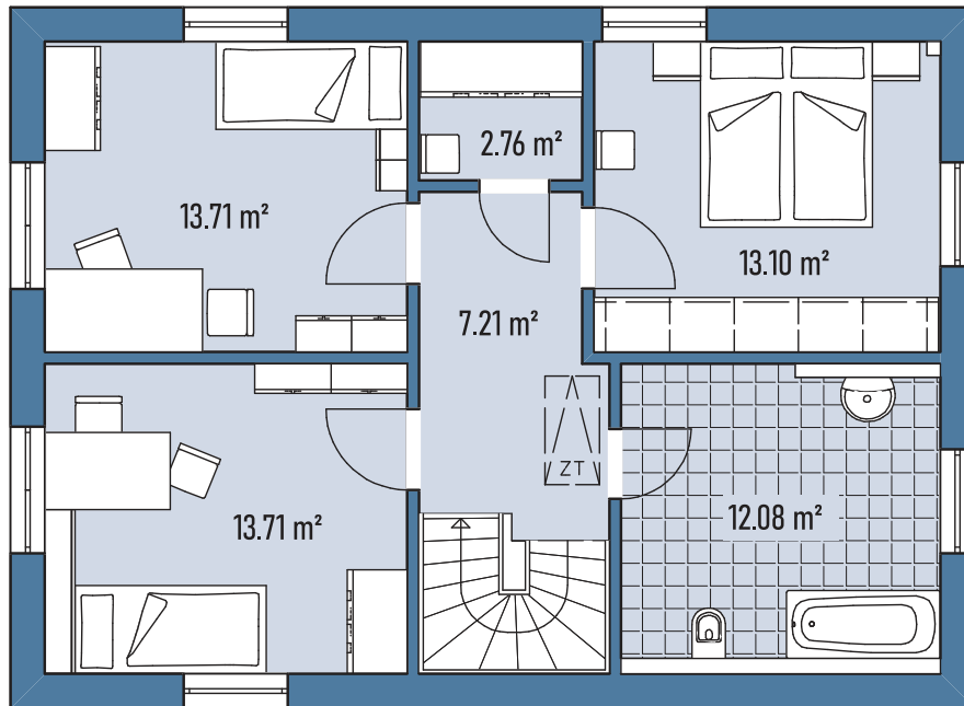
Grundriss DG
