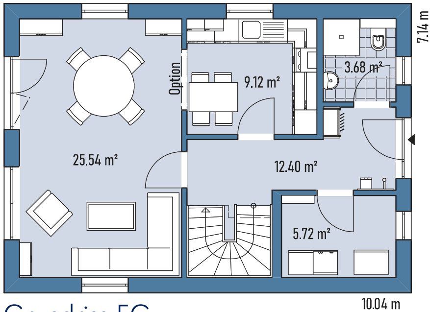
Grundriss EG
