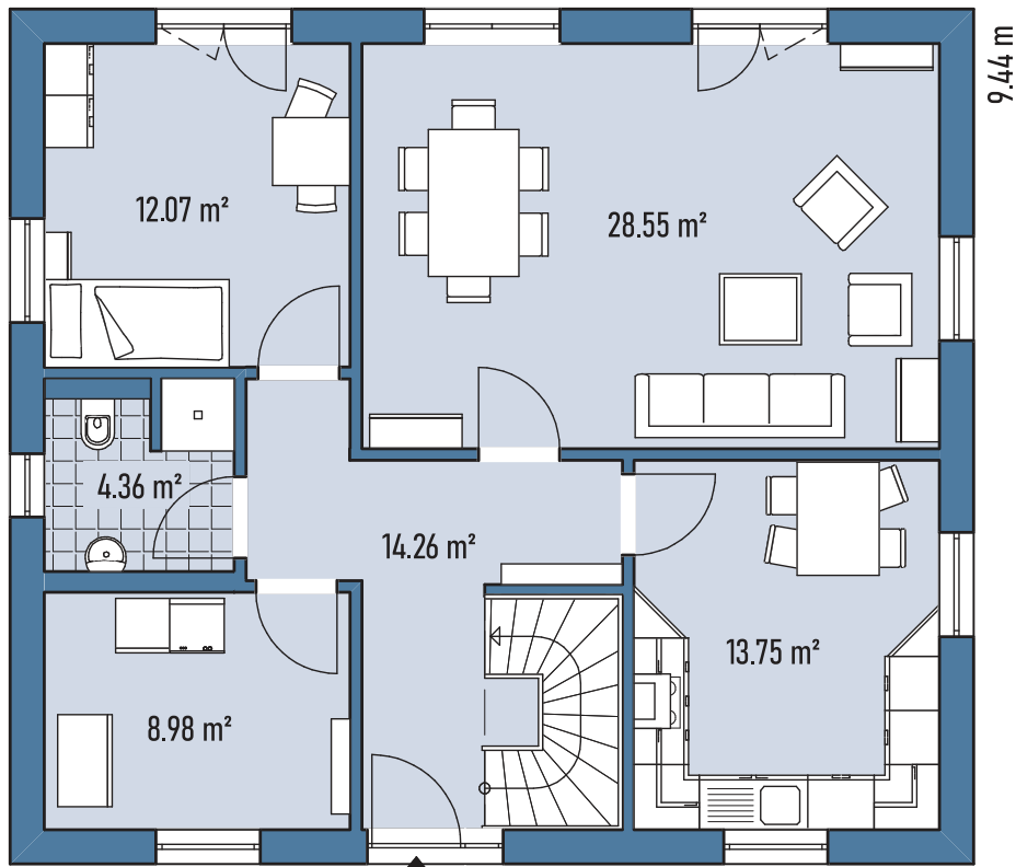
Grundriss EG
