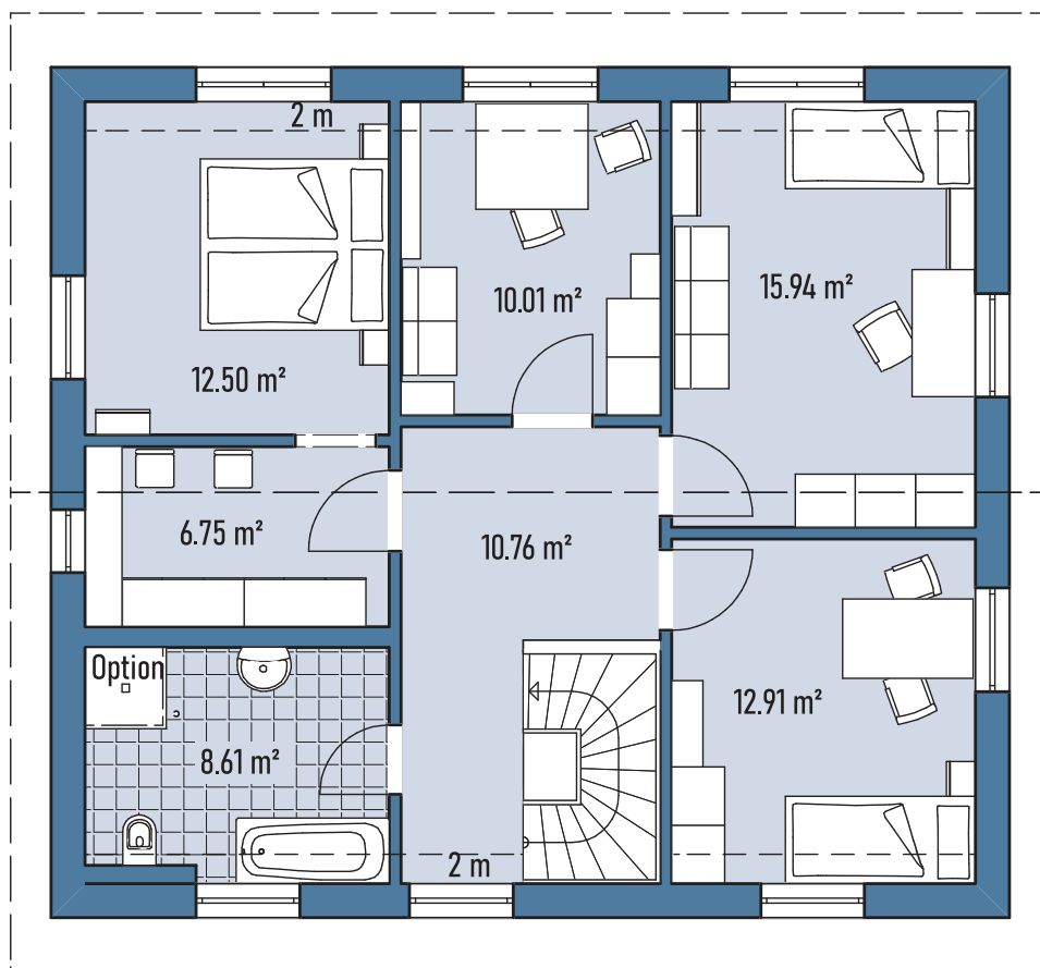
Grundriss DG
