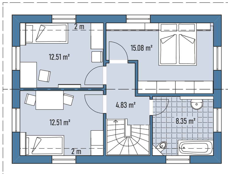
Grundriss DG
