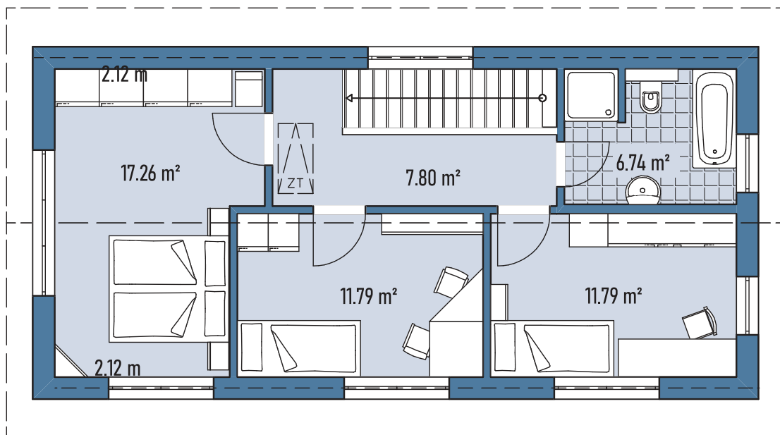
Grundriss DG
