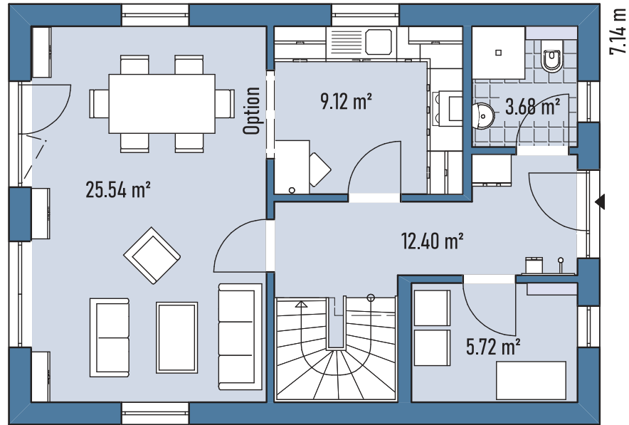
Grundriss EG
