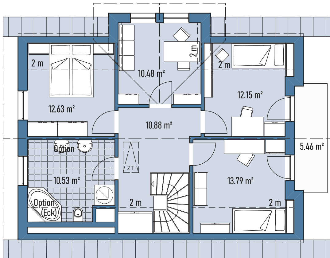
Grundriss DG
