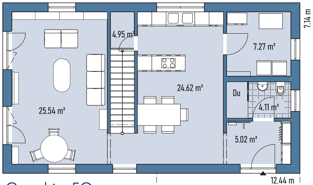
Grundriss EG
