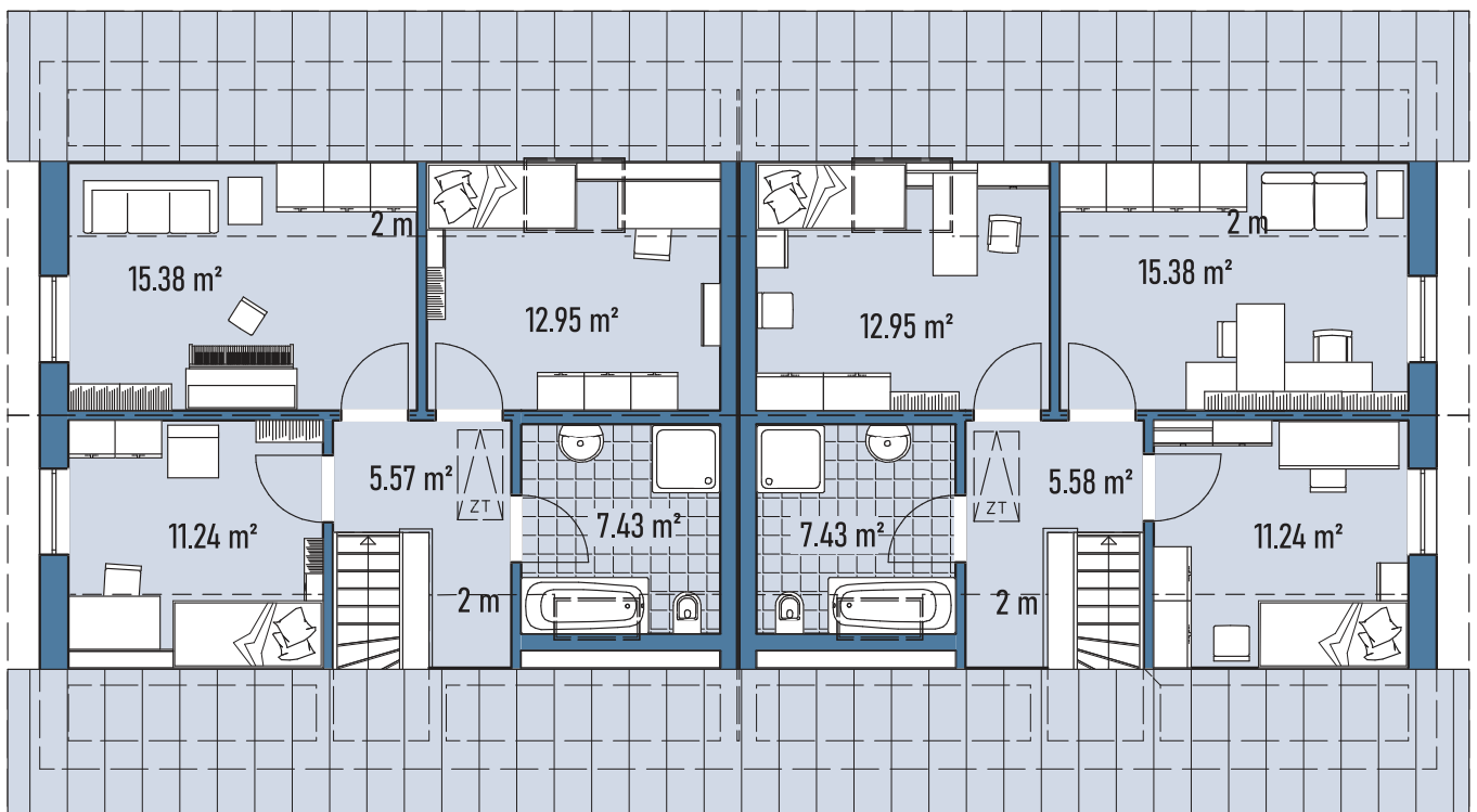
Grundriss DG
