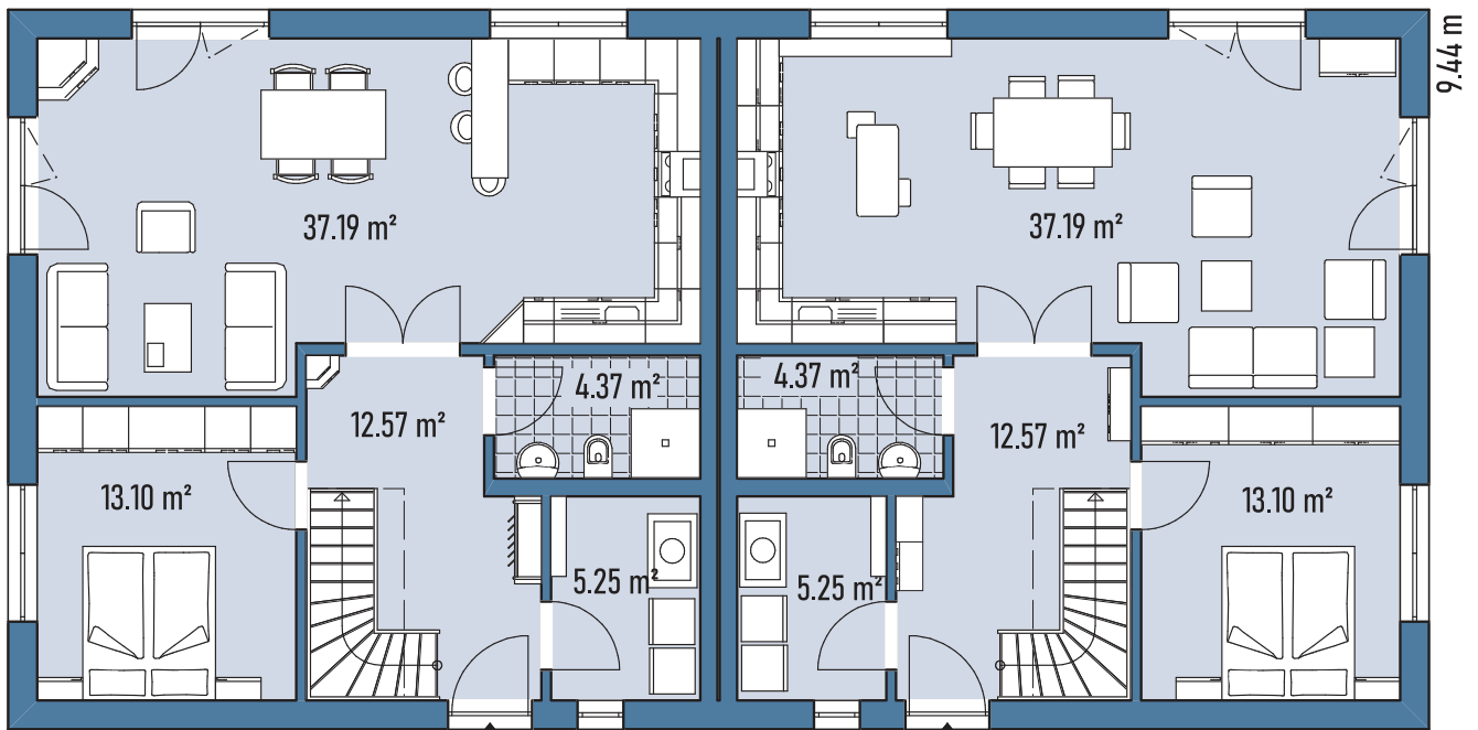
Grundriss EG
