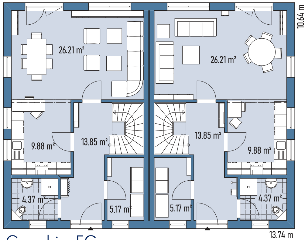
Grundriss EG
