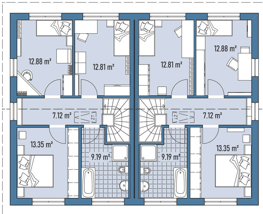
Grundriss DG
