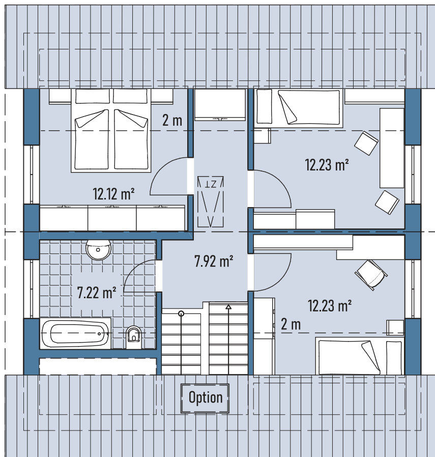
Grundriss DG
