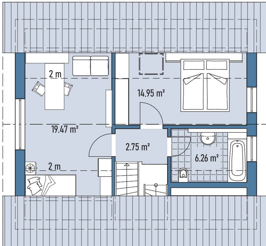
Grundriss DG
