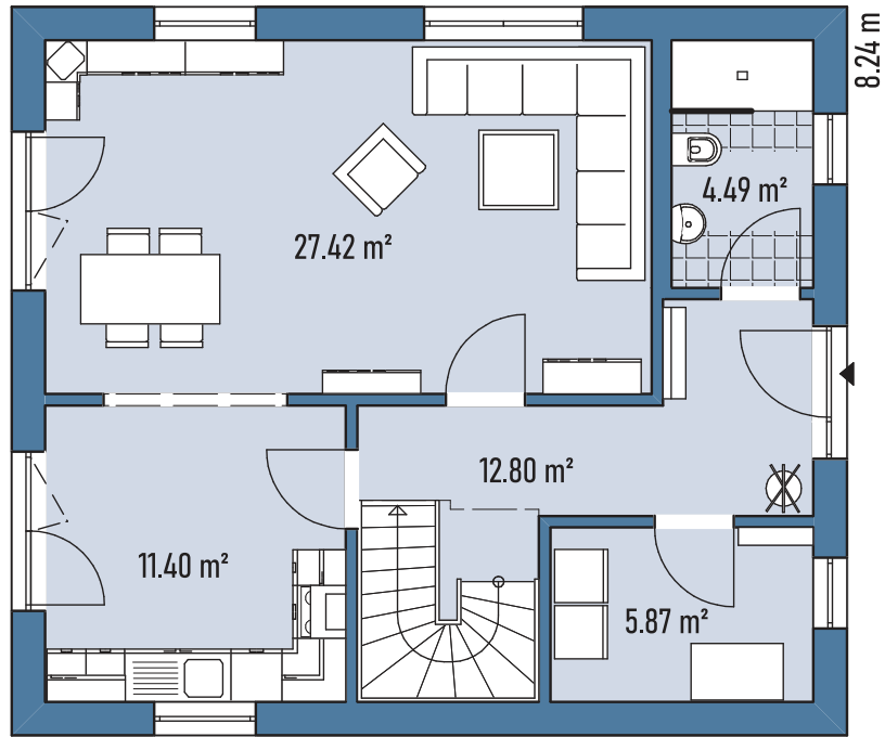
Grundriss EG
